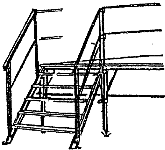
Escalier monté
